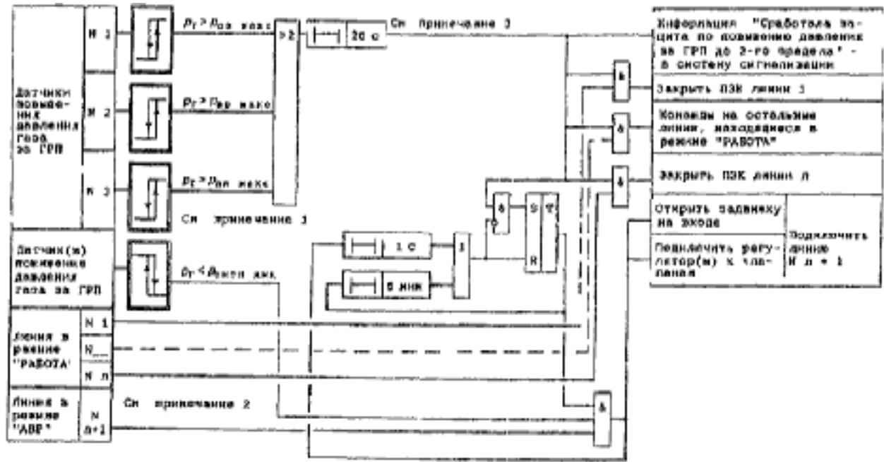
Рис. 2. Структурная схема защиты по повышению давления газа ГРП до 2-го предела для ГРП, на которых установлены ПЗК.
