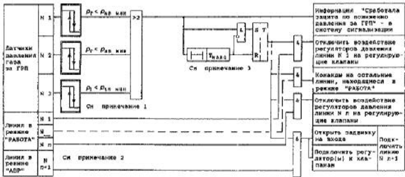
Рис. 4. Структурная схема защиты по повышению давления газа ГРП.
