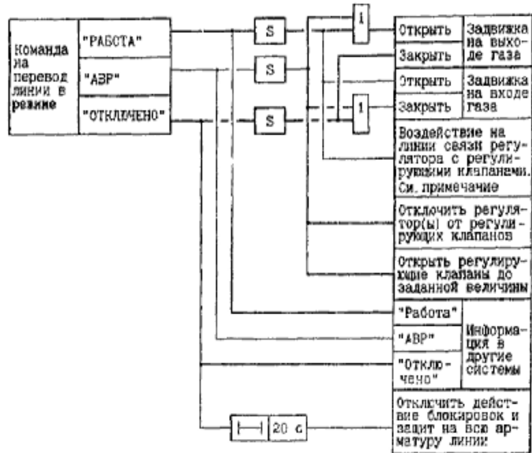
Рис. 5. Структурная схема блокировки по переводу линии редуцирования газа в новый режим.
