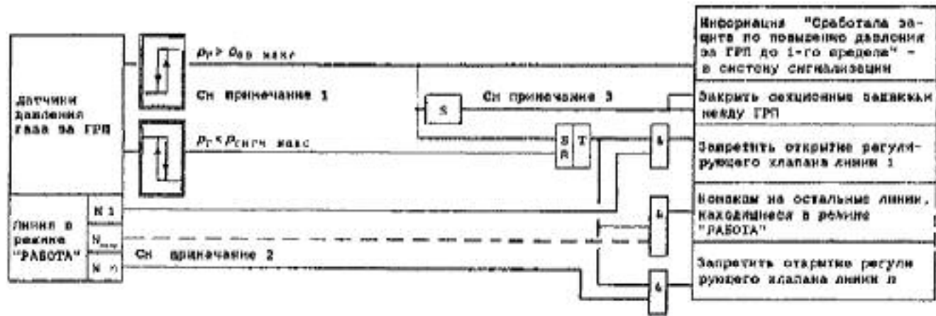
Рис. 1. Структурная схема защиты по повышению давления газа ГРП до 1-го предела.
