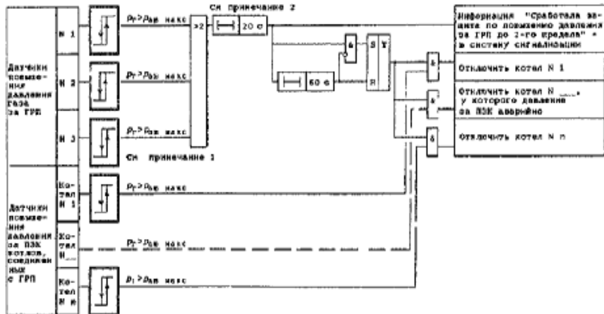
Рис. 3. Структурная схема защиты по повышению давления газа за ГРП, где все элементы газопроводов до ПЗК котлов рассчитаны на давление газа до ГРП.
