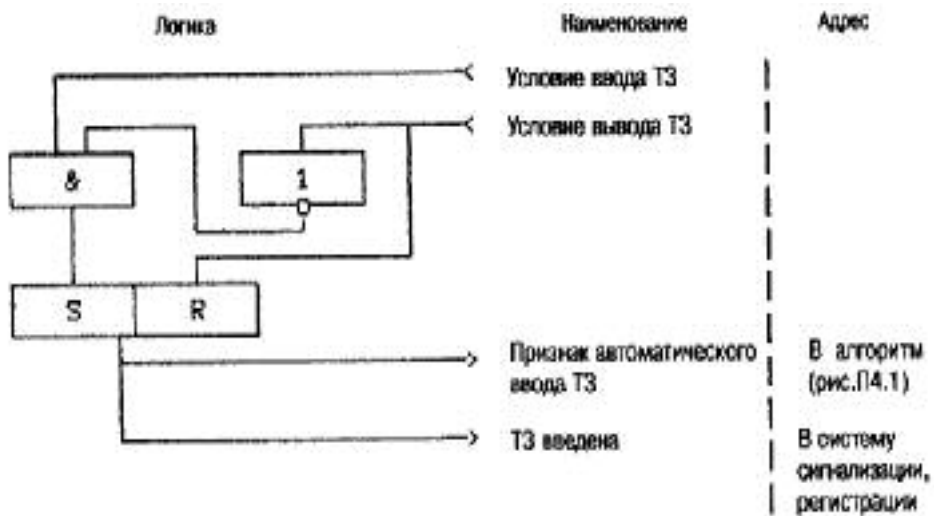
Рис. П4.2. Формирование признака автоматического ввода ТЗ
