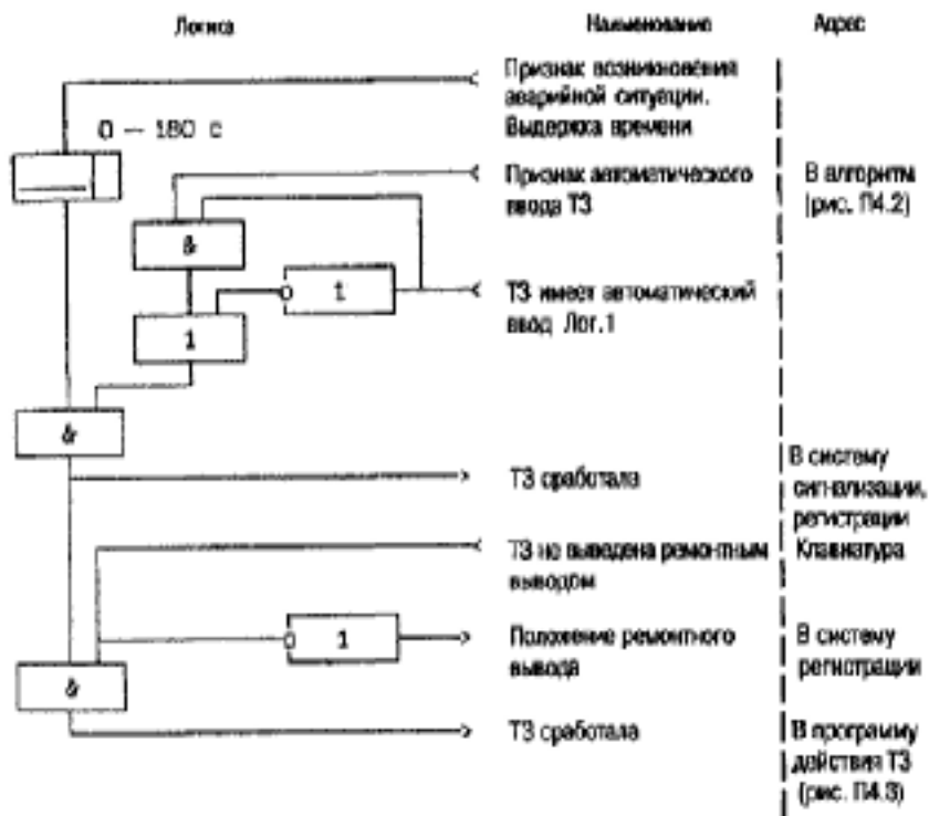
Рис. П4.1. Формирование условий срабатывания ТЗ
