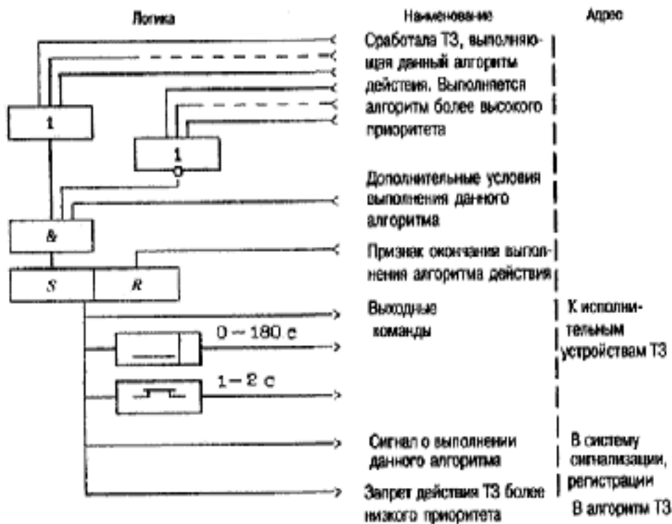
Рис. П4.3. Алгоритм действия ТЗ
