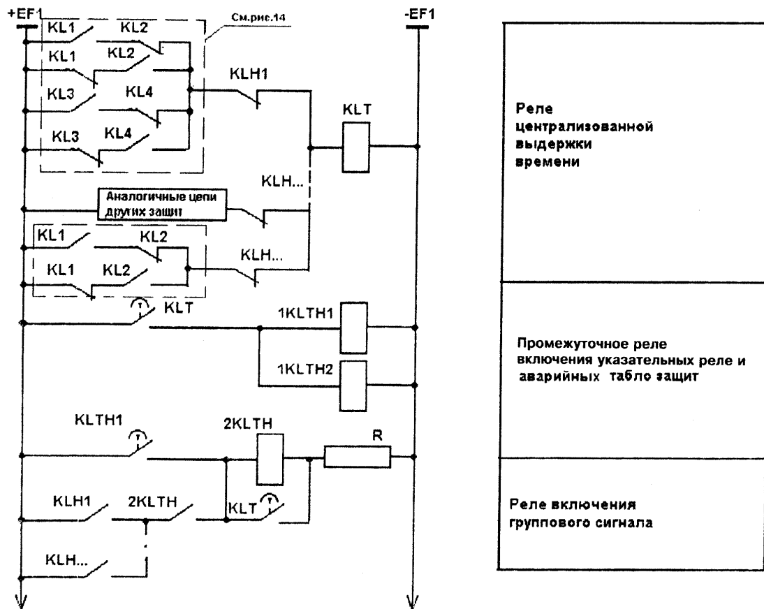
Рис. 21. Электрическая схема организации сигнала "Сработал один из двух датчиков защиты" на реле (2 листа)
