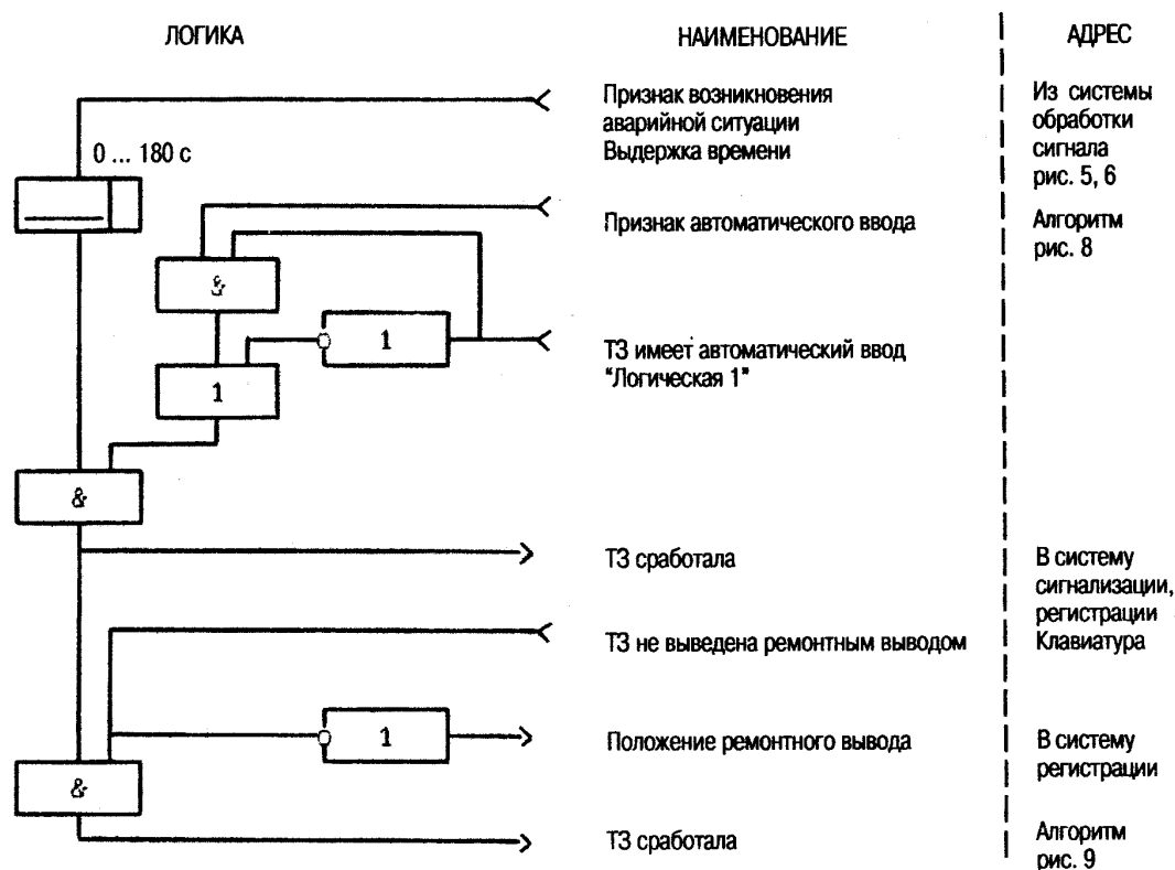
Рис. 7. Алгоритм формирования условий срабатывания ТЗ
