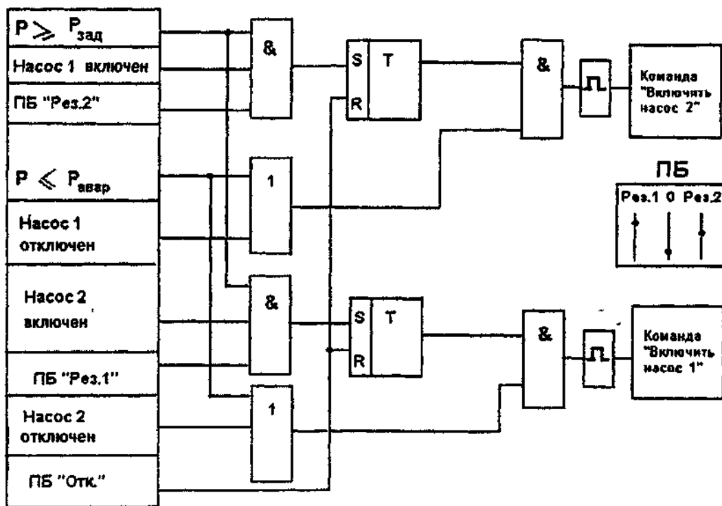
Рис. 11. Алгоритм АВР двух насосов с общим переключателем и контролем давления в напорной магистрали
