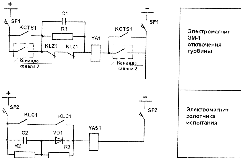
Рис. 23. Организация электрической схемы опробования электромагнита отключения турбины при двухканальной схеме защит (3 листа)
