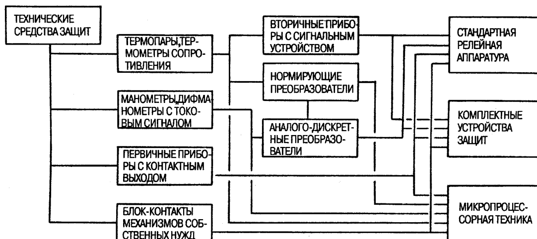
Рис. 4. Классификация защит по техническим средствам
