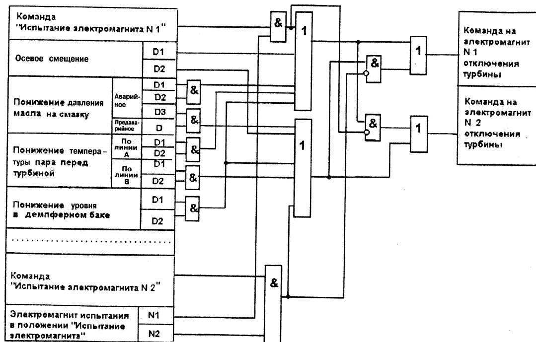
Рис. 10 Алгоритм организации двухканальной схемы защит
