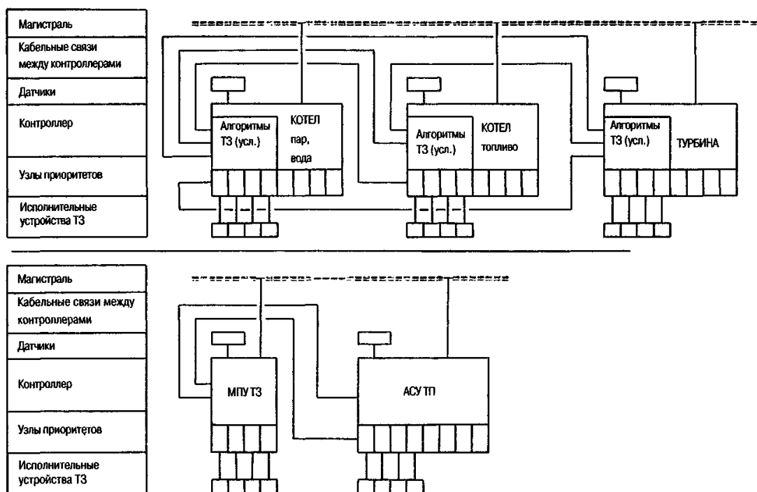
Рис. 20. Связи подсистемы ТЗ с другими для разных вариантов ее выполнения на МПТ
