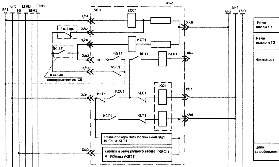
Рис. 19. Электрическая схема ТЗ турбины на УКТЗ (5 листов)
