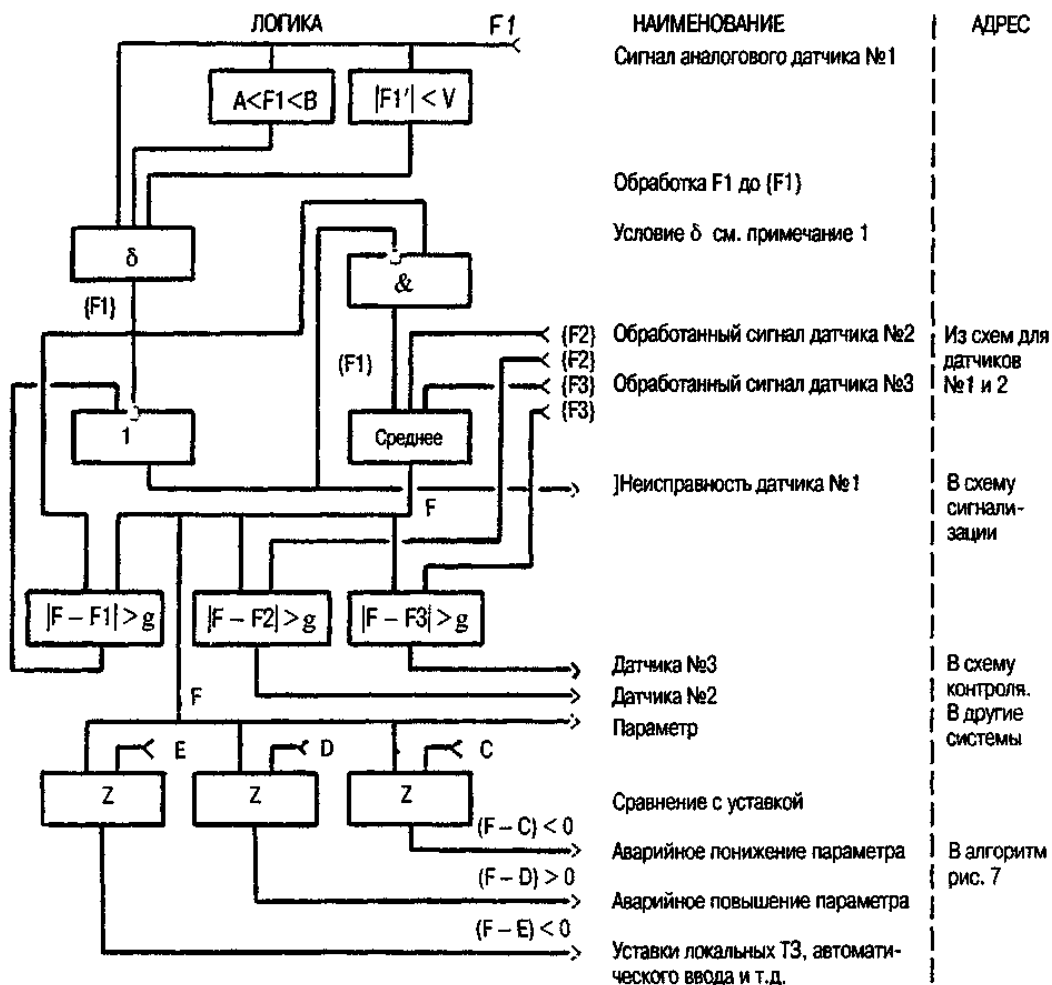
Рис. 6. Алгоритм обработки аналоговых сигналов датчиков одного параметра
