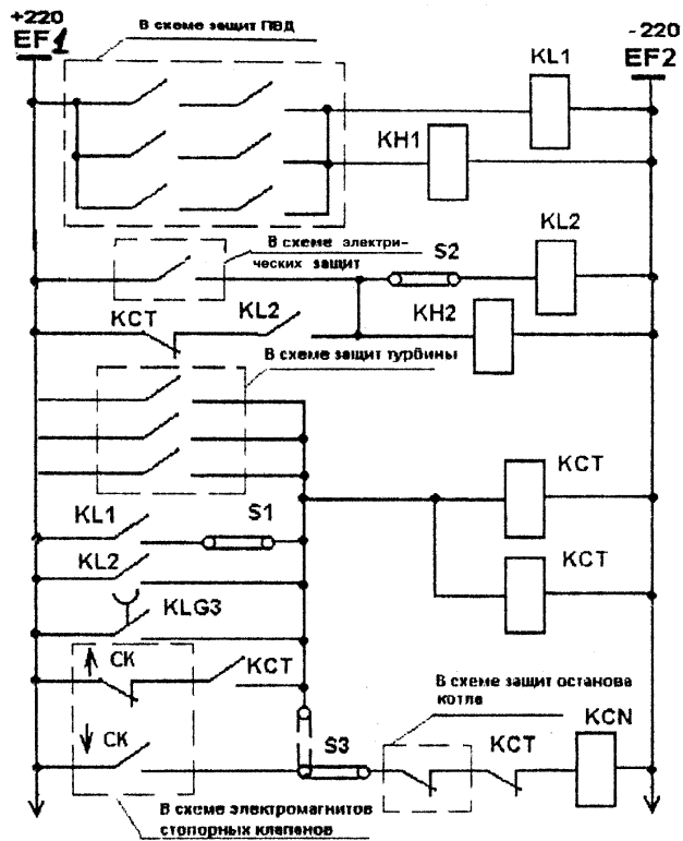
Рис. 13. Электрическая схема общеклочных защит (2 листа):
