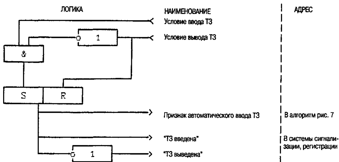
Рис. 8. Алгоритм формирования признака автоматического ввода ТЗ
