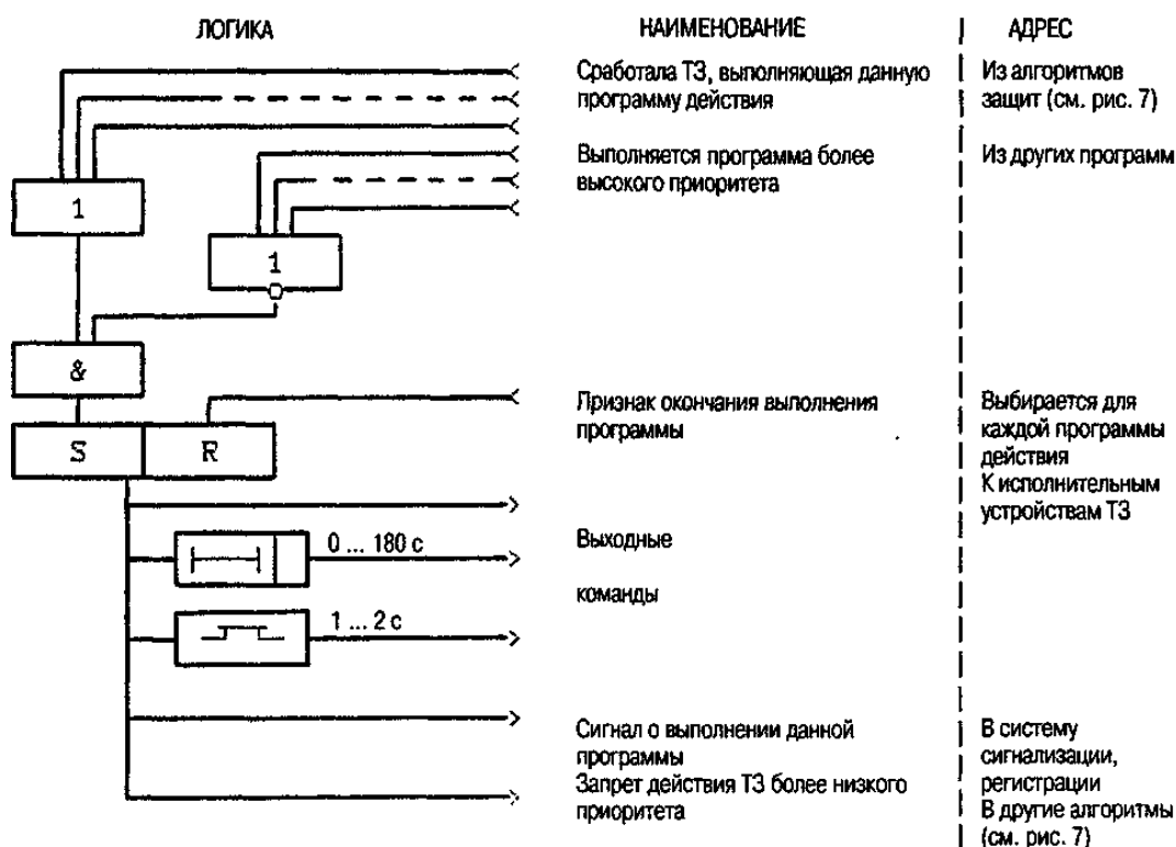
Рис. 9. Алгоритм программы действия ТЗ
