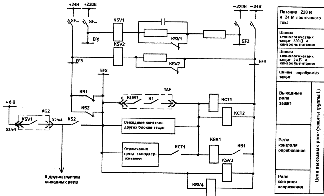
Рис. 24. Организация электрической схемы опробования ТЗ на УКТЗ (7 листов)
