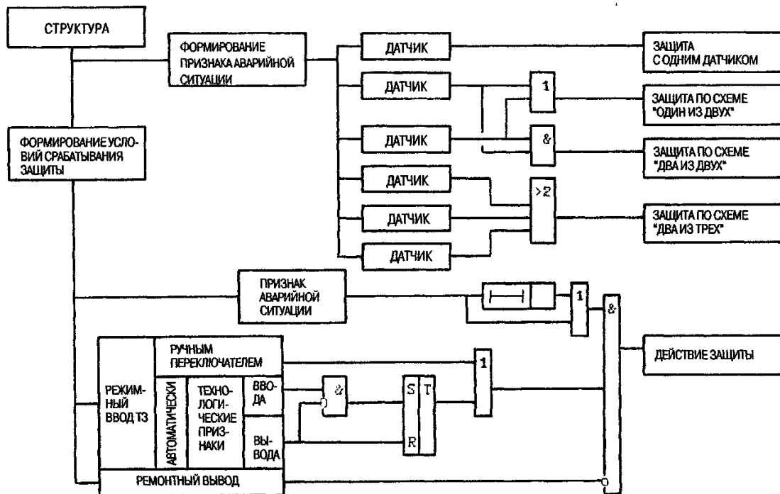
Рис. 2. Классификация защит по количеству датчиков и структуре
