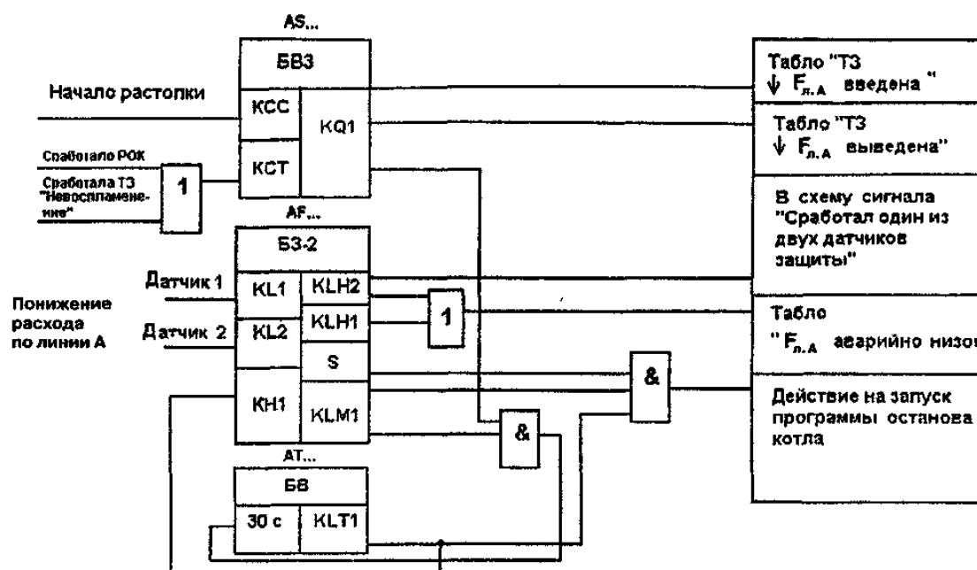
Рис. 18. Структурная схема организации защиты на блоках УКТЗ
