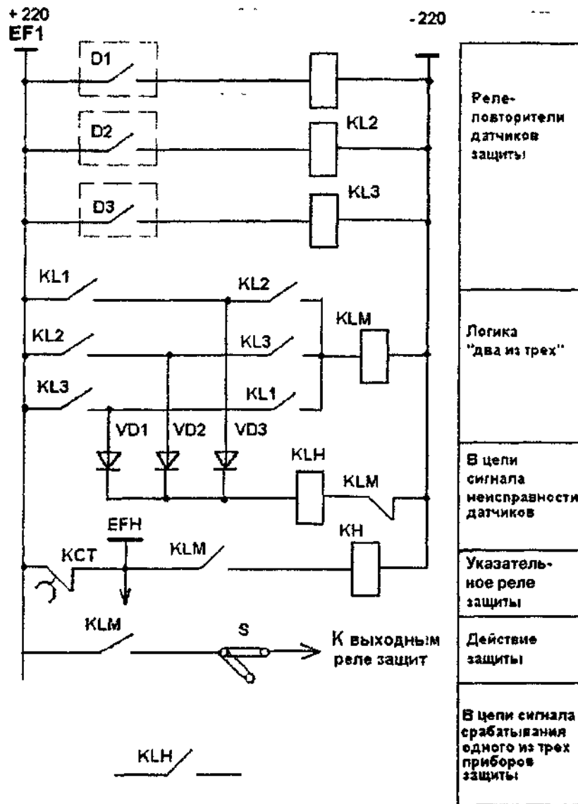
Рис. 15. Электрическая схема защиты по схеме "два из трех"
