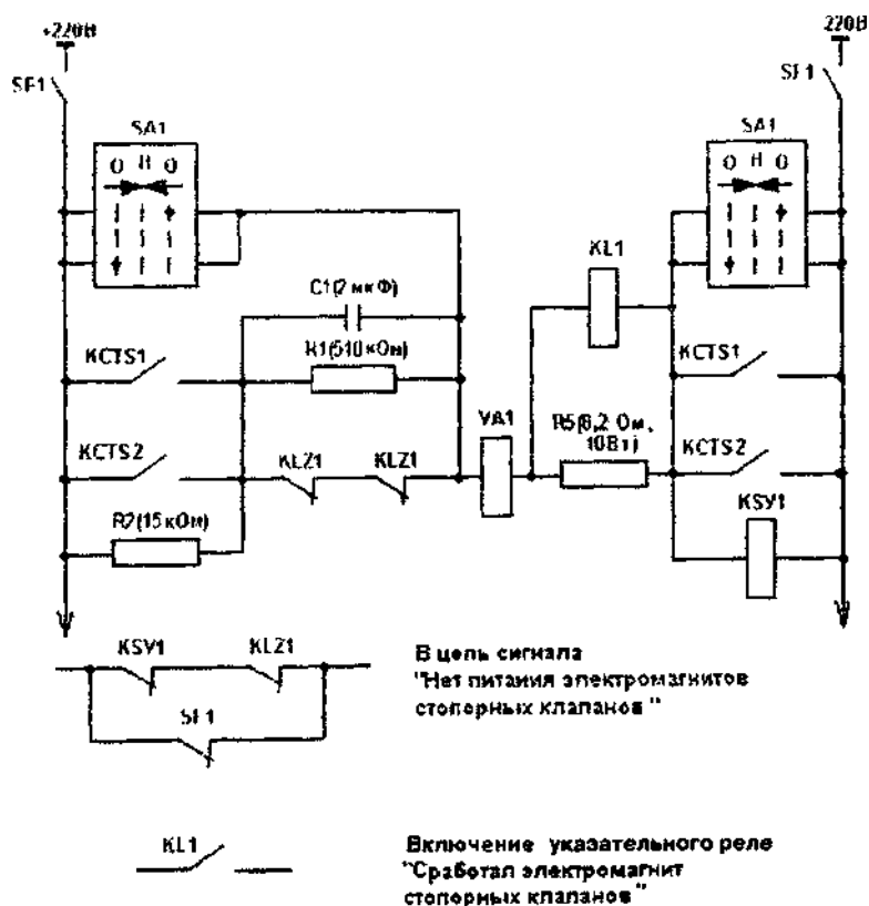
Рис. 17. Электрическая схема управления электромагнитами стопорных клапанов турбины
