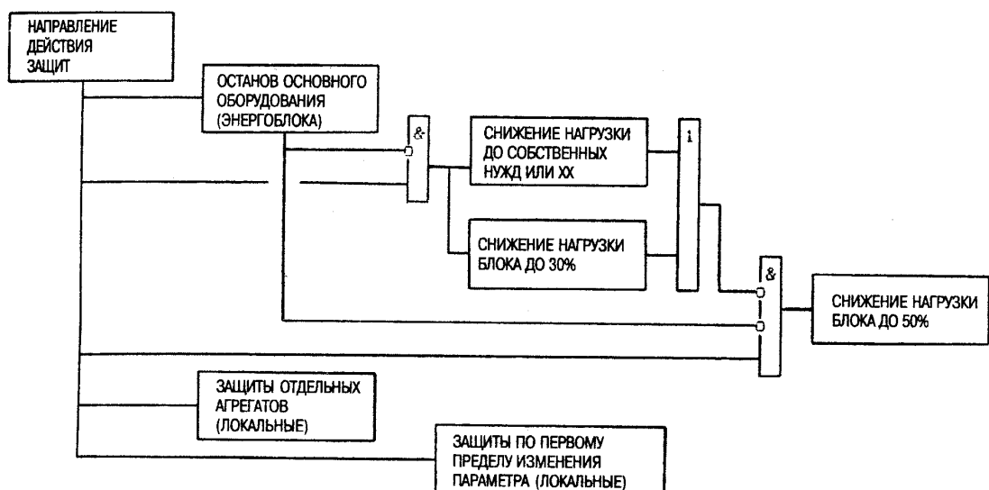
Рис. 1. Классификация защит по направлению действия
